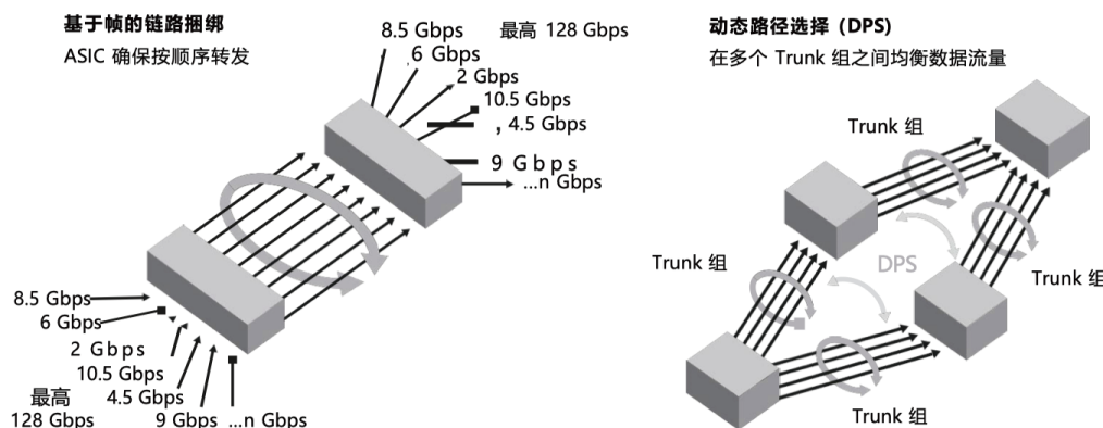
图 1. 动态路径选择(DPS)可补充UNIS ISL链路捆绑，在多个捆绑链路组之间高效地路由数据
